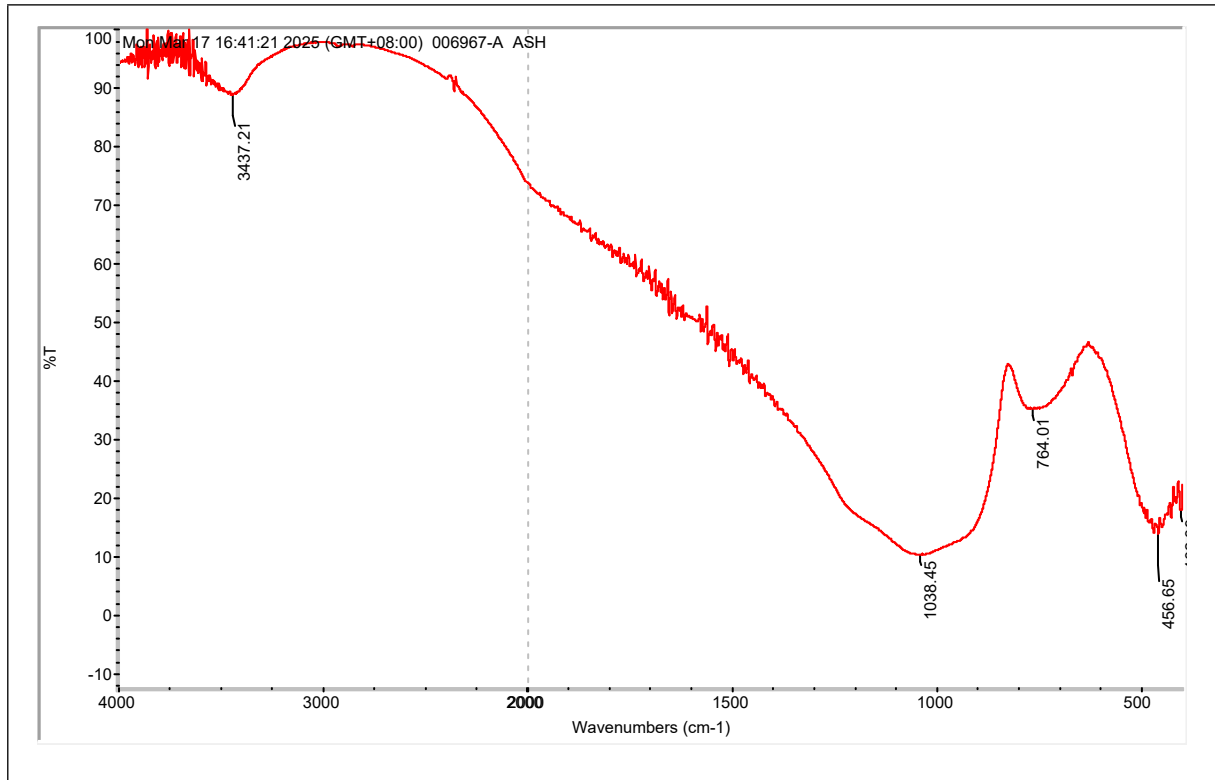
图 2: 灼烧残余的 FTIR 谱图
