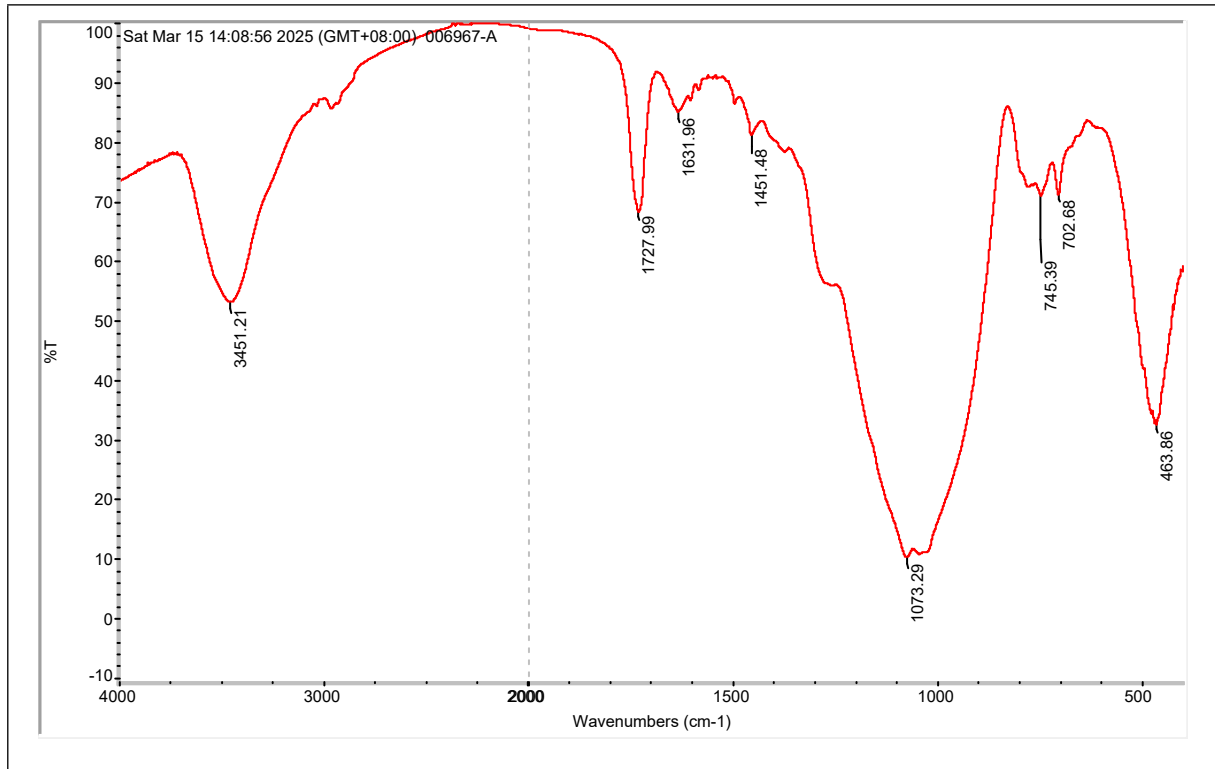
图 1: 原样的 FTIR 谱图
